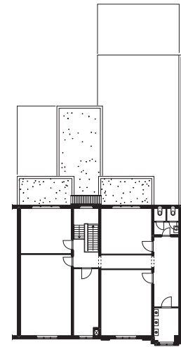
nieuwe situatie 2 e verdieping
